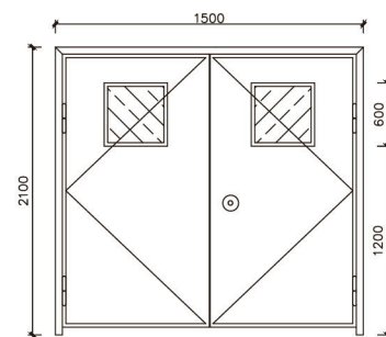
双开门示意图
